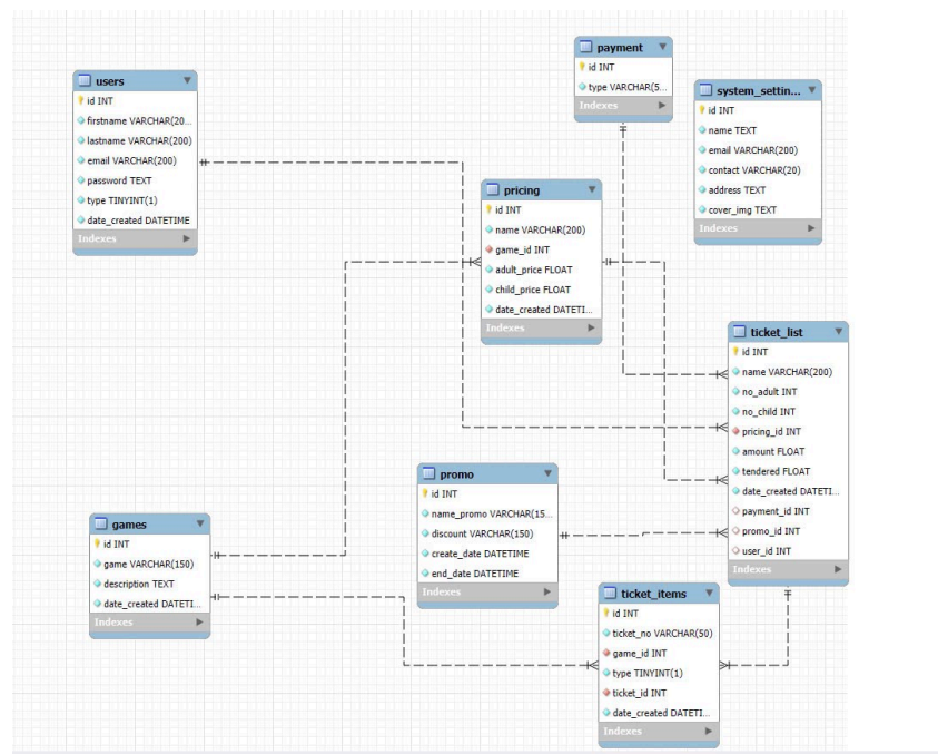
Hình 3.2: Lược đồ quan hệ chuẩn 3NF
